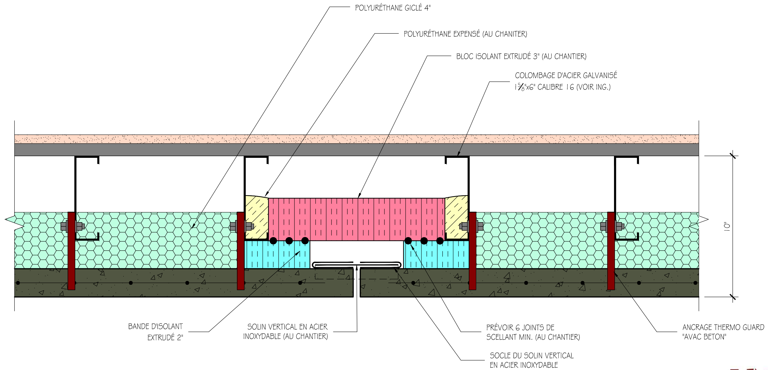
DÉTAIL DE JOINT VERTICAL ENTRE DEUX PANNEAUX ÉCHELLE: NAE
